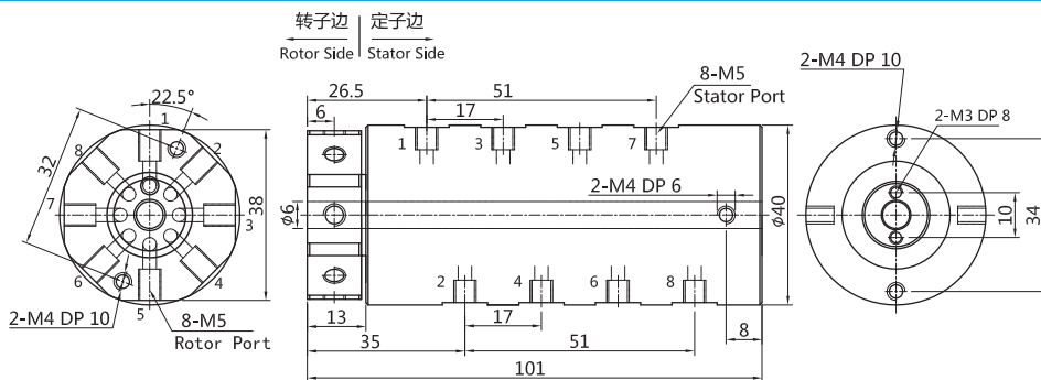
3008004 (8进8出, 4mm气管, 纯气动旋转接头) 尺寸图
