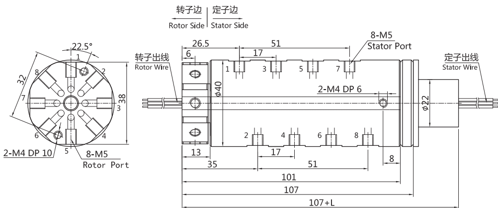
3008004 (8进8出,4mm气管) +6~36路信号系列尺寸图 (适用于电磁阀与感应开关)
